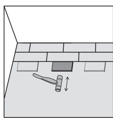
Position of the planks: Correct, Position of the planks: Incorrect, Position of the planks: Incorrect. Posición de las planchas: Correcta, Posición de las planchas: Incorrecta, Posición de las planchas: Incorrecta.
